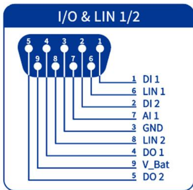
图 1-4 引脚定义 (LIN、I/O)
