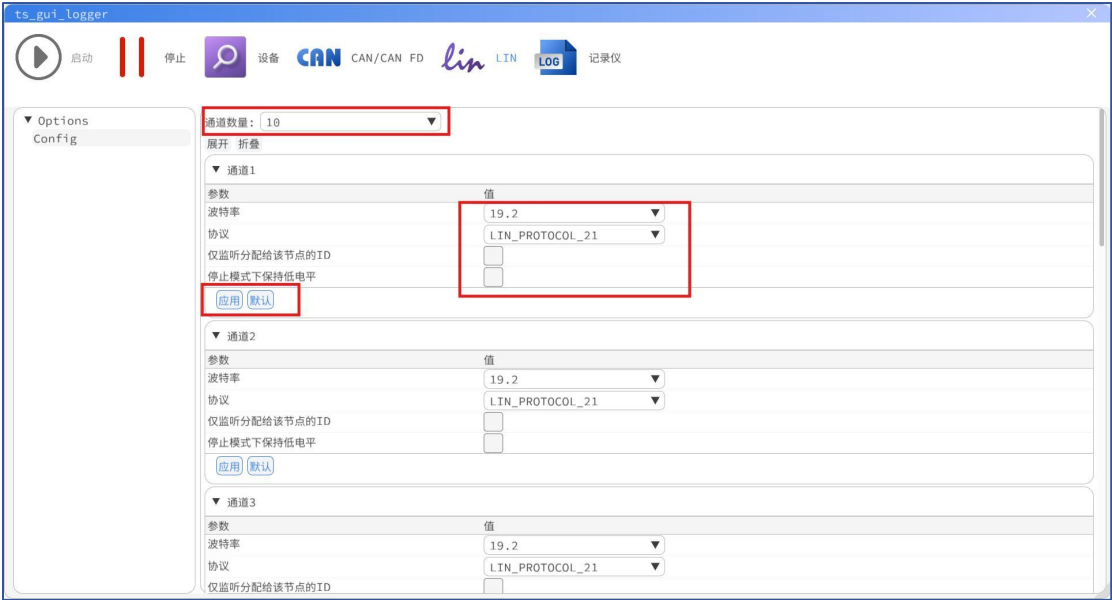
图 2-28 LIN 通道配置
