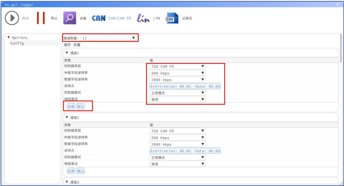
图 2-27 CAN 通道配置
