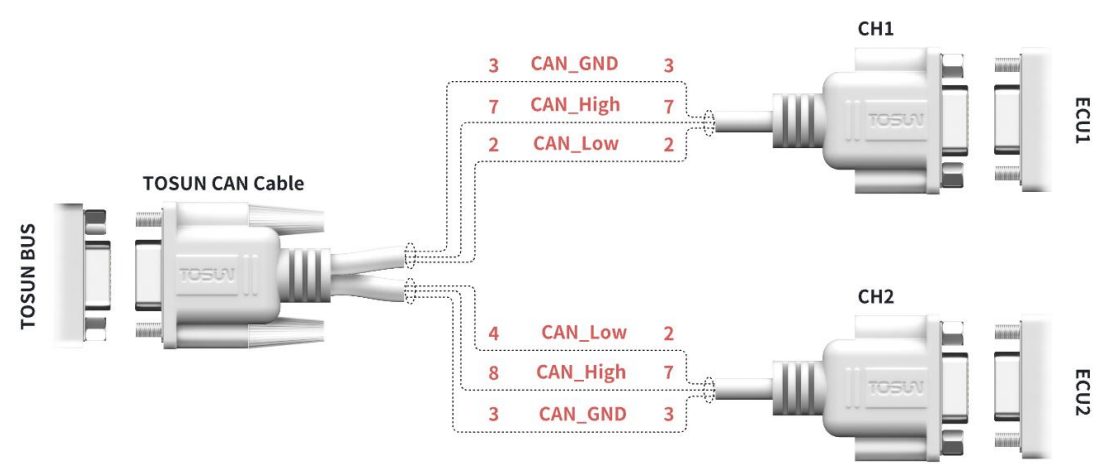
图 2-5 DB9 母一分二公头信号线（CAN）
