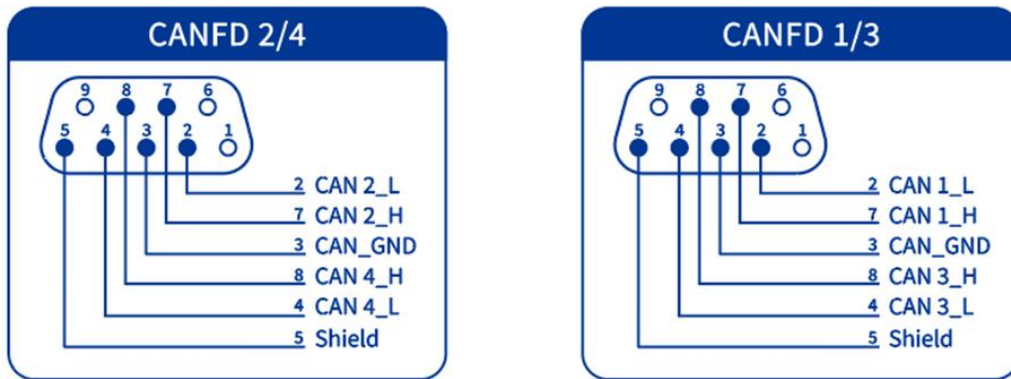
图 1-3 引脚定义 (CAN FD)
