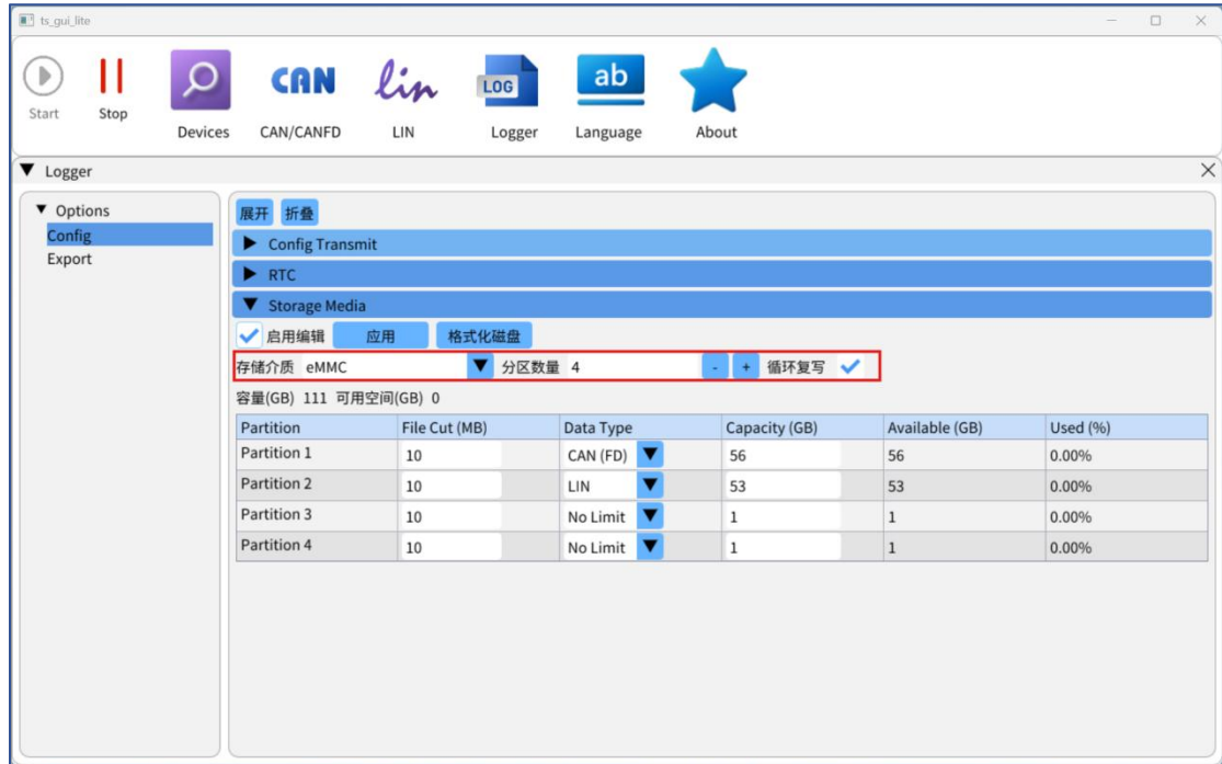
图 2-33 eMMC 配置
