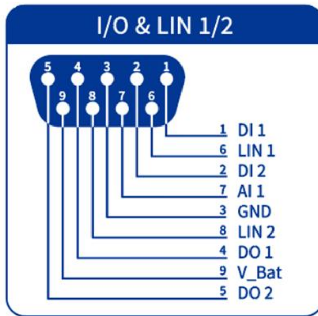
图 1-4 引脚定义 (LIN、I/O)
