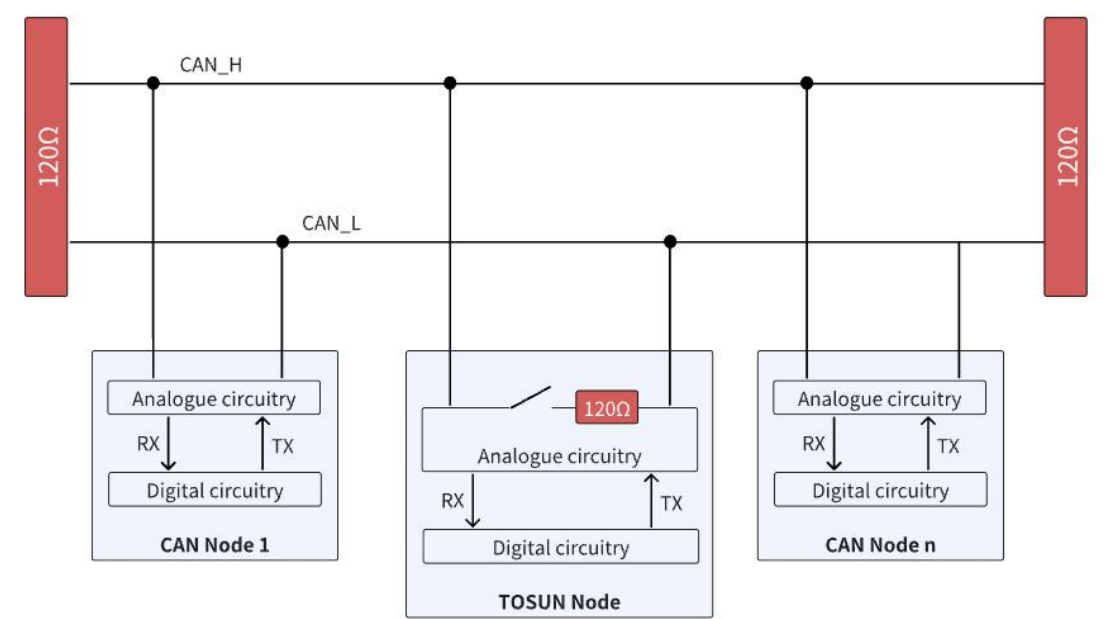
图 2-5 接入 CAN 总线
