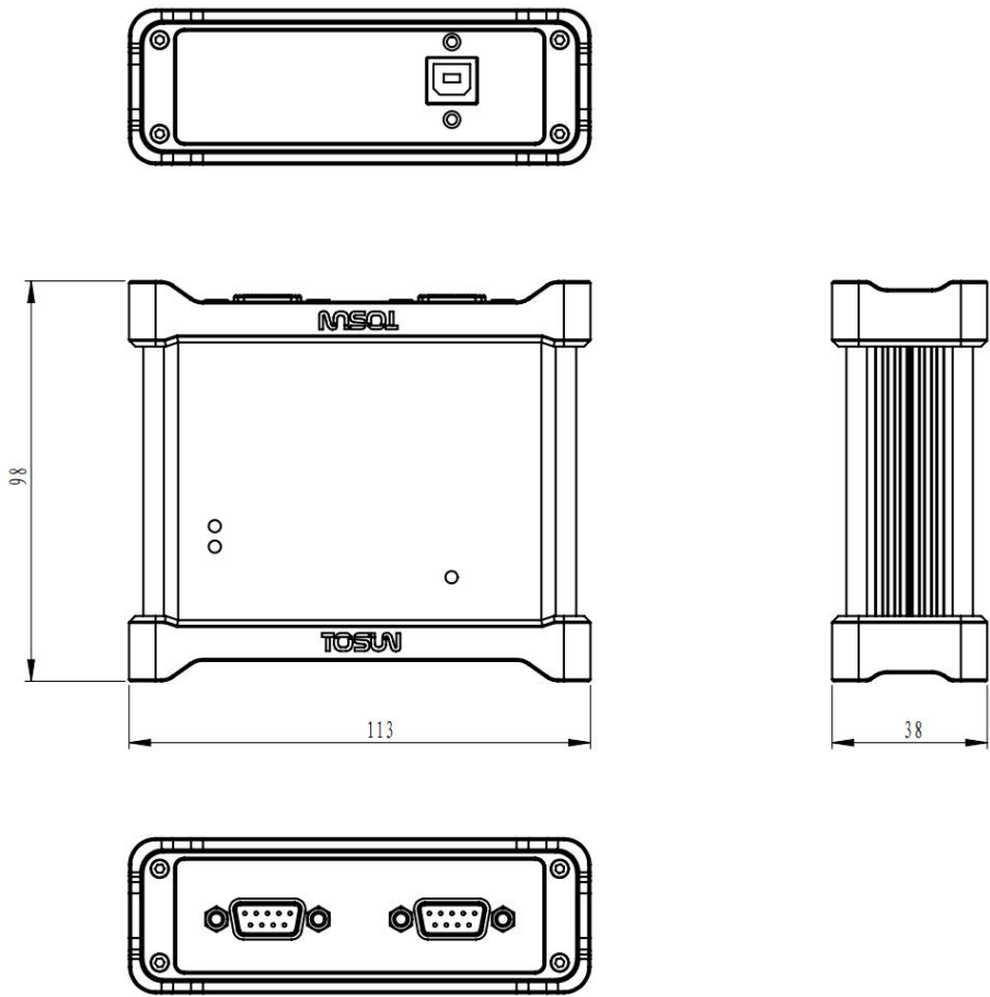
图 1-1 机械尺寸
