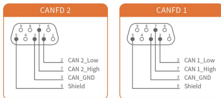
图 1-3 引脚定义（CAN FD）
