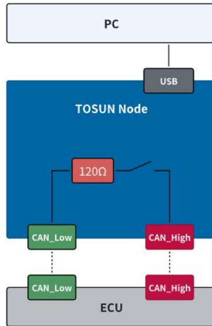
图 2-4 使用 CAN
