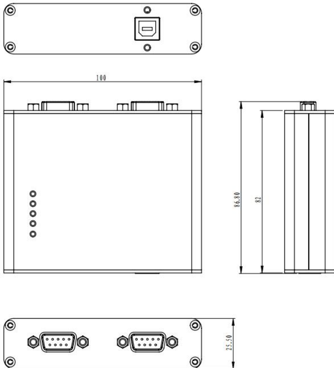
图 1-1 机械尺寸
