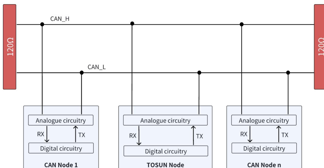
图 2-2 接入 CAN 总线
