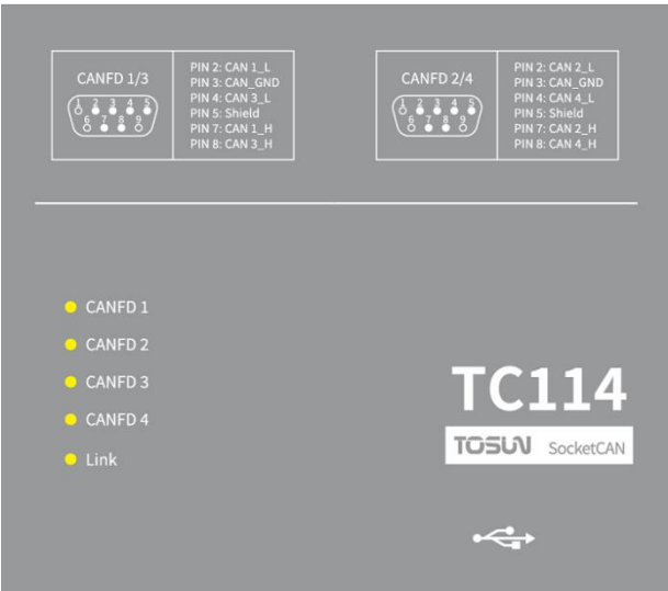
图 1-2 产品正面贴膜
