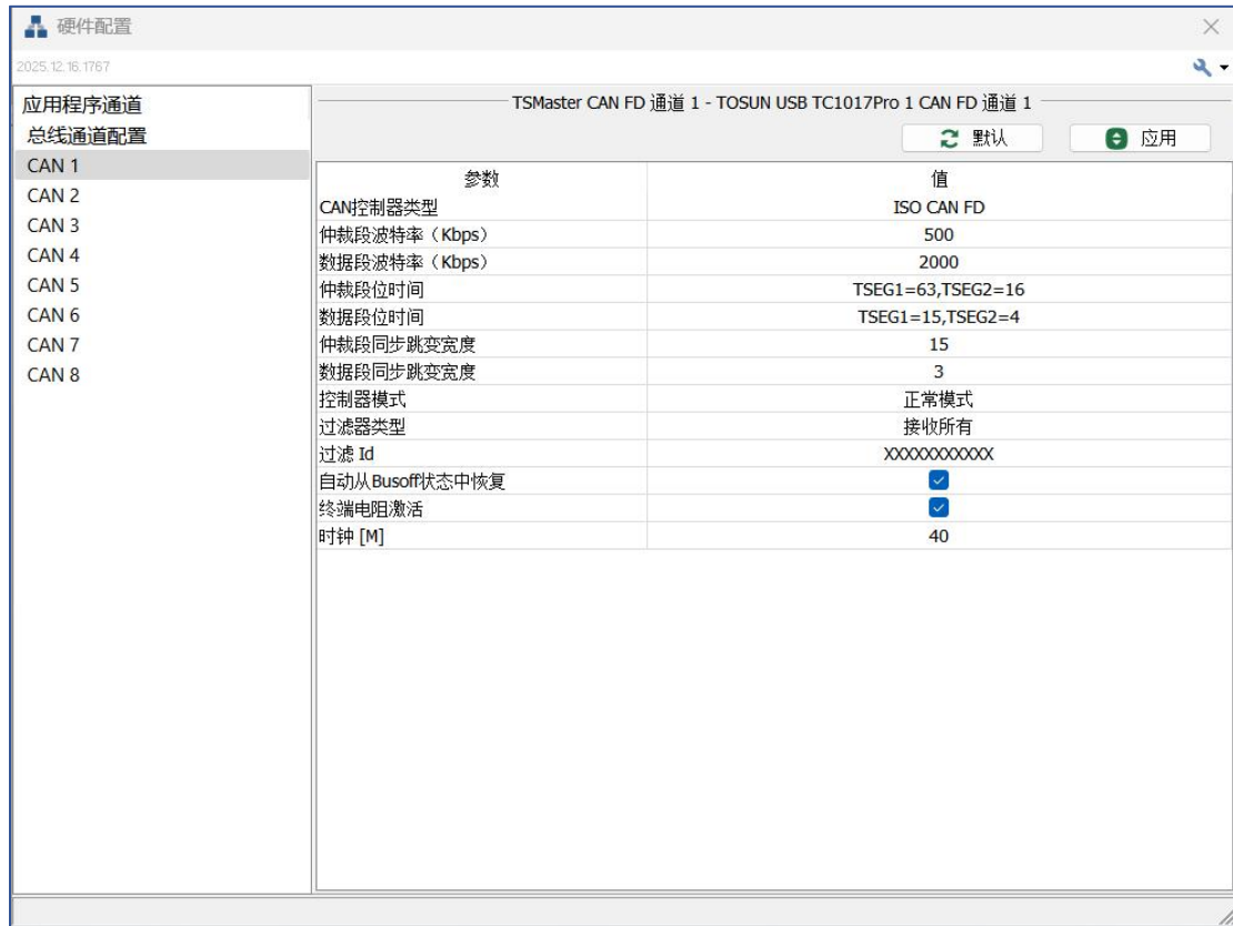
图 2-6 通道配置 (CAN)
