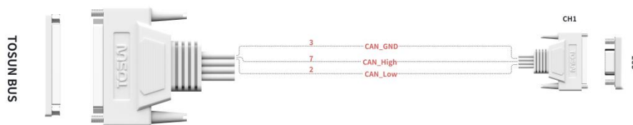
图 2-10 DB37 母转 8 公信号线 (CAN)
