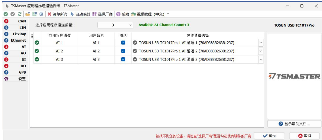
图 2-3 AI 通道选择
