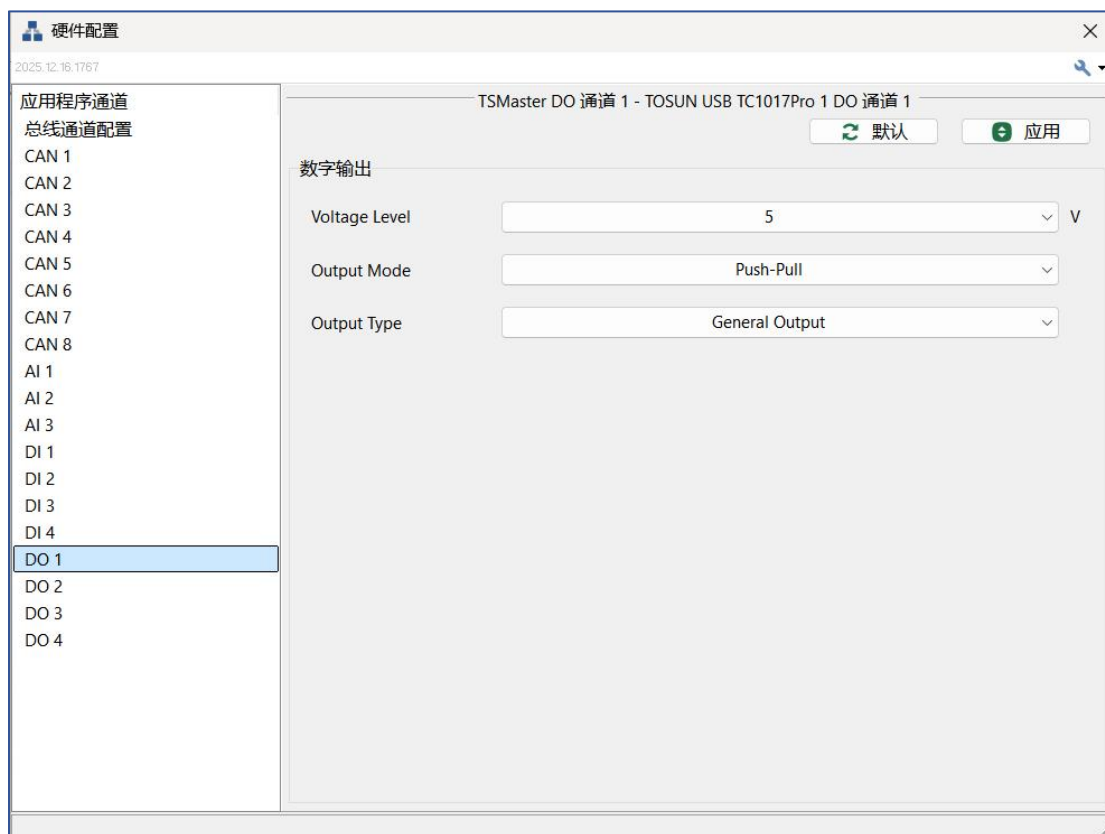
图 2-9 DO 通道配置 (I/O)
