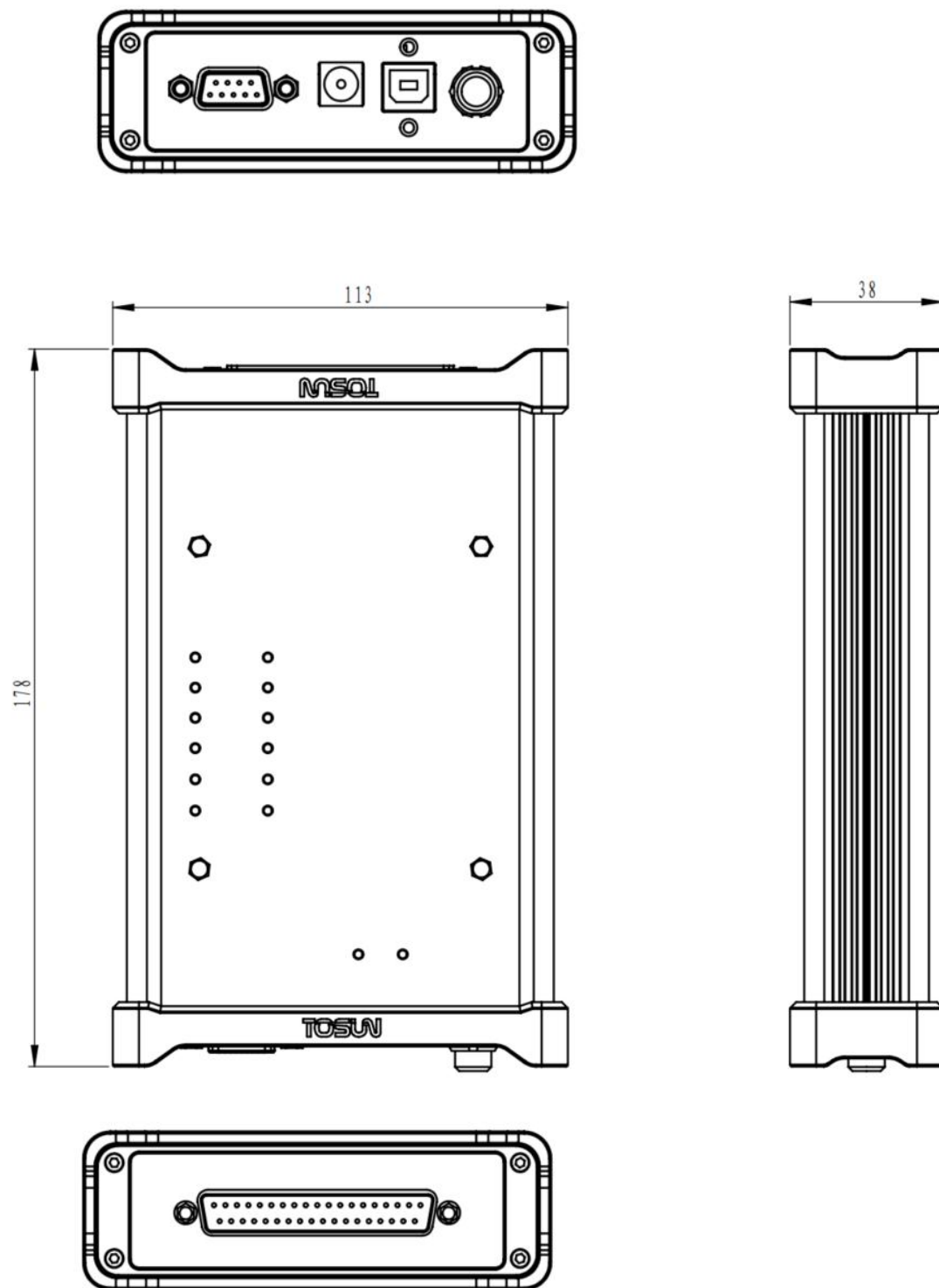
图 1-1 机械尺寸
