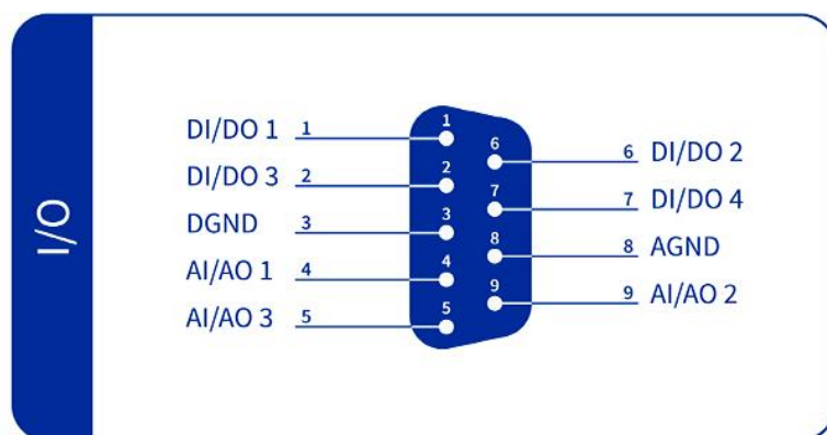
图 1-5 引脚定义 (I/O)
