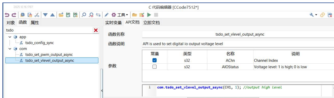
图 2-28 使用 C 小程序配置 DO 输出高低电平
