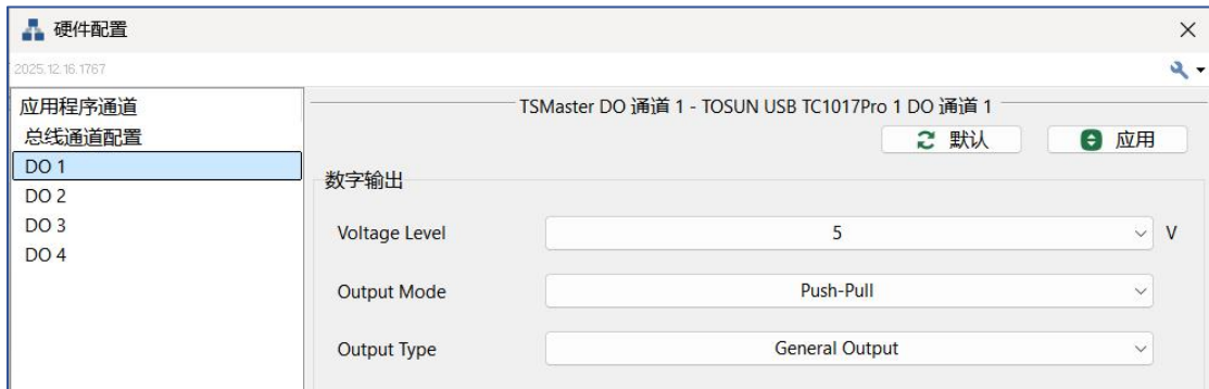
图 2-26 使用硬件配置 DO 参数
