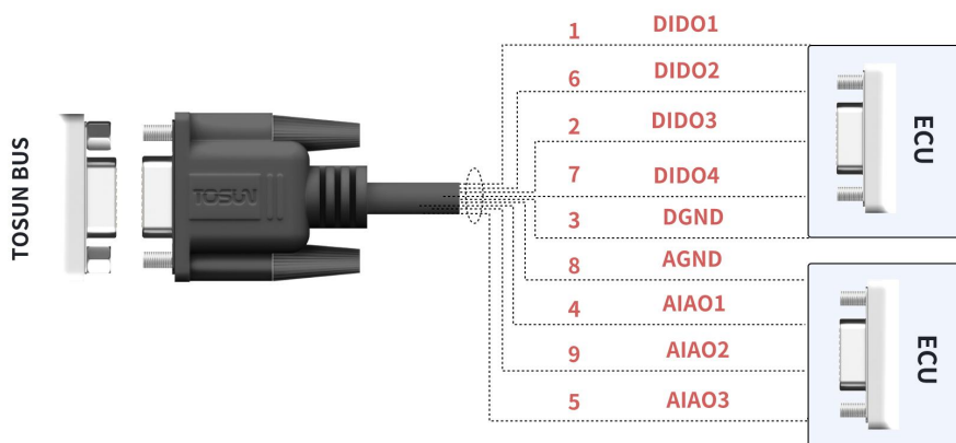
图 2-13 模拟量数字量接口 DB9 公头线束
