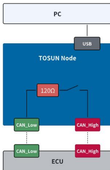
图 2-11 使用 CAN
