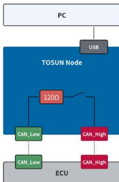
图 2-3 使用 CAN
