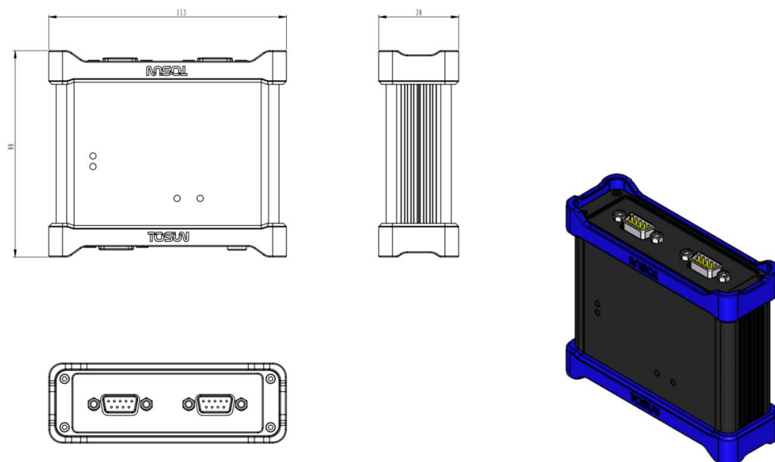
图 1-1 机械尺寸
