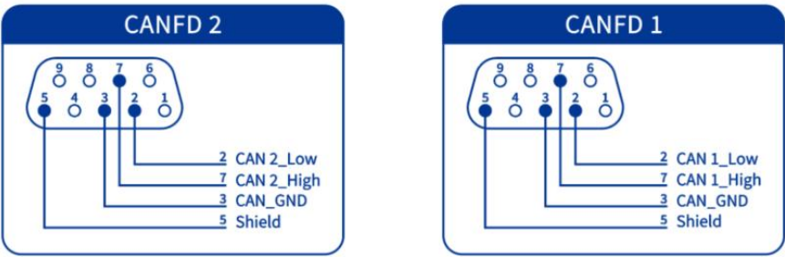
图 1-3 引脚定义（CAN FD）
