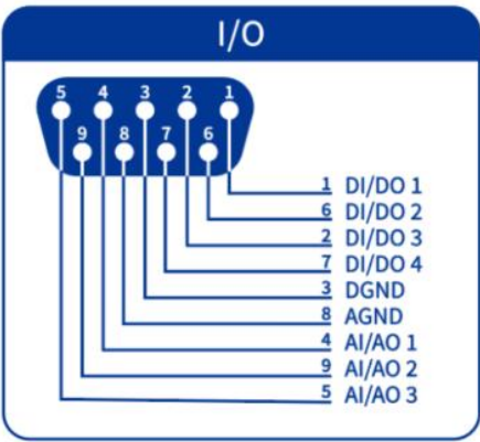
图 1-5 引脚定义（I/O）
