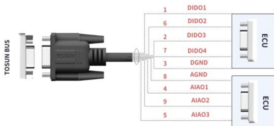
图 2-5 I/O 接线图
